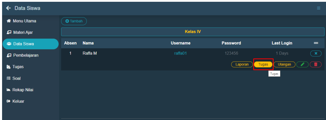
Gambar 26. Tombol Tugas
