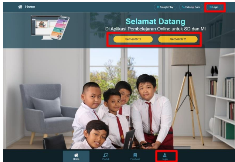
Gambar 5. Menu Login
