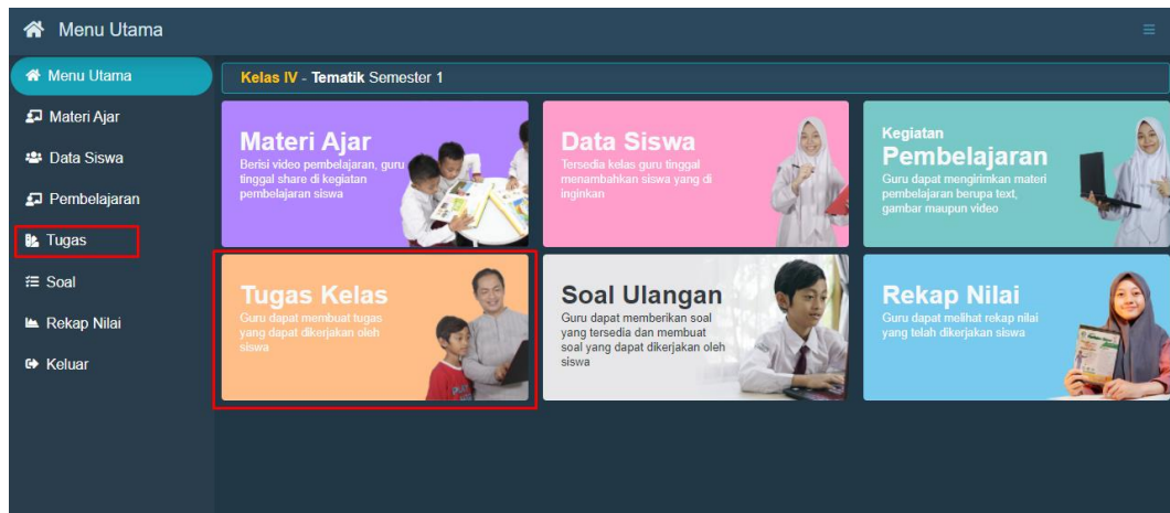
Gambar 43. Menu Tugas
