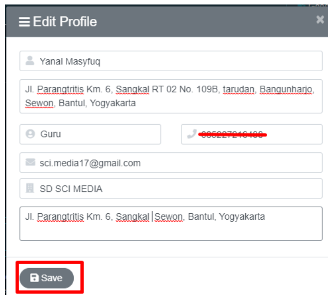
Gambar 9. Merubah profile
