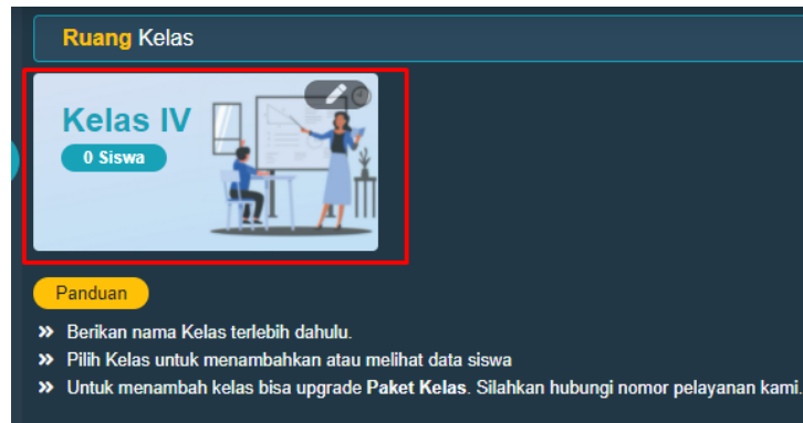
Gambar 17. Icon Kelas
