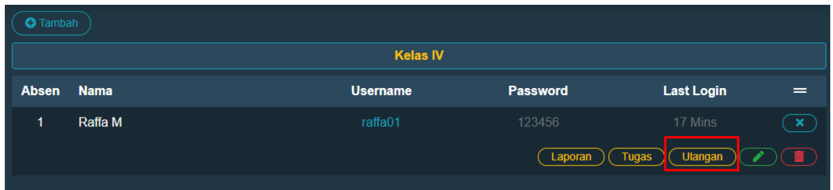
Gambar 31. Tombol Ulangan
