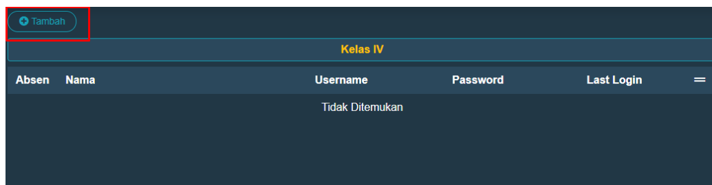
Gambar 18. Tambah siswa
