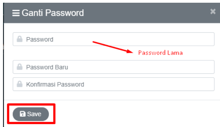
Gambar 12. Mengganti Password
